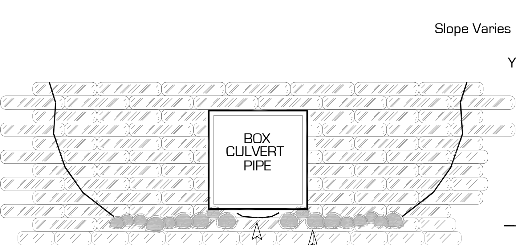
ELEVATION
