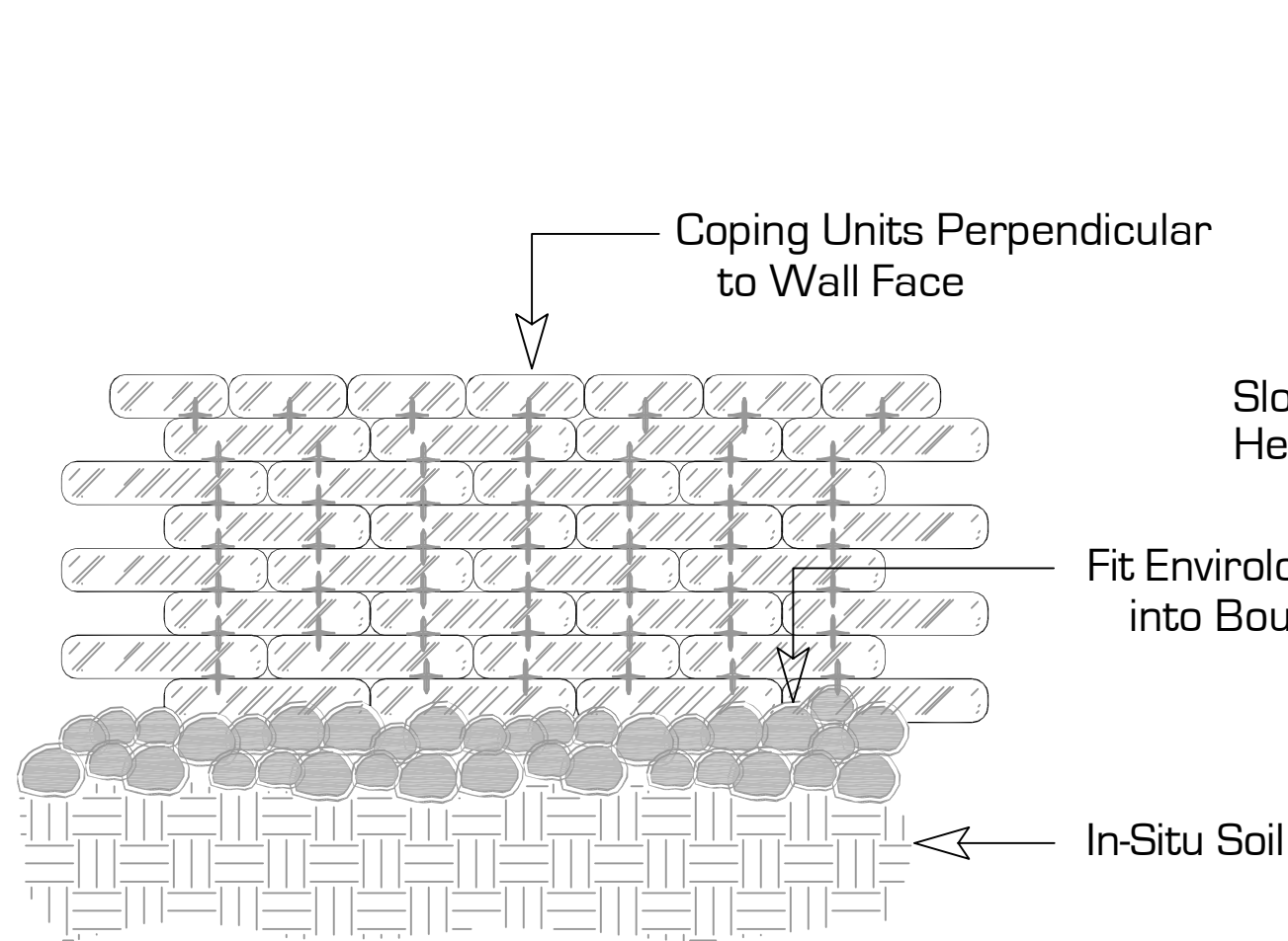
ELEVATION
